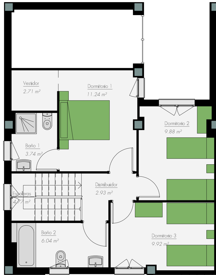
VIVIENDA TIPO 1 Planta alta
